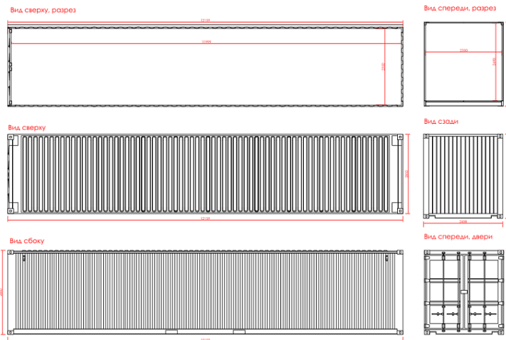
Планировка контейнера 40ft
