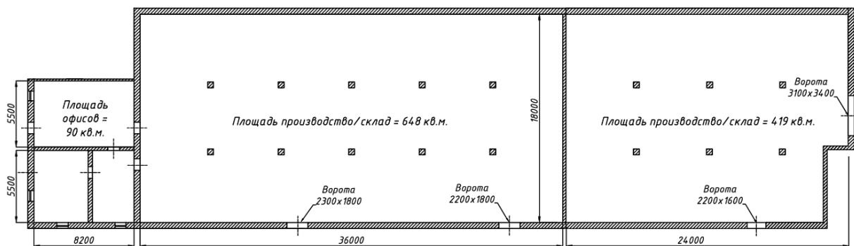
Планировка лит. 3
